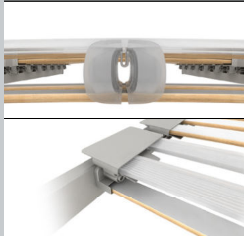
ERGO-GUIDE in der Schulterzone
